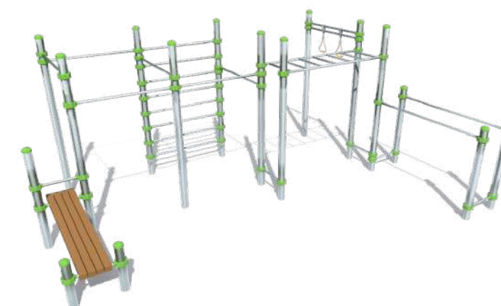
2 ОБОРУДОВАНИЕ WORKOUT Производитель: Феникс, артикул: WRK 14 Размеры: 5900x4800x2700 мм
