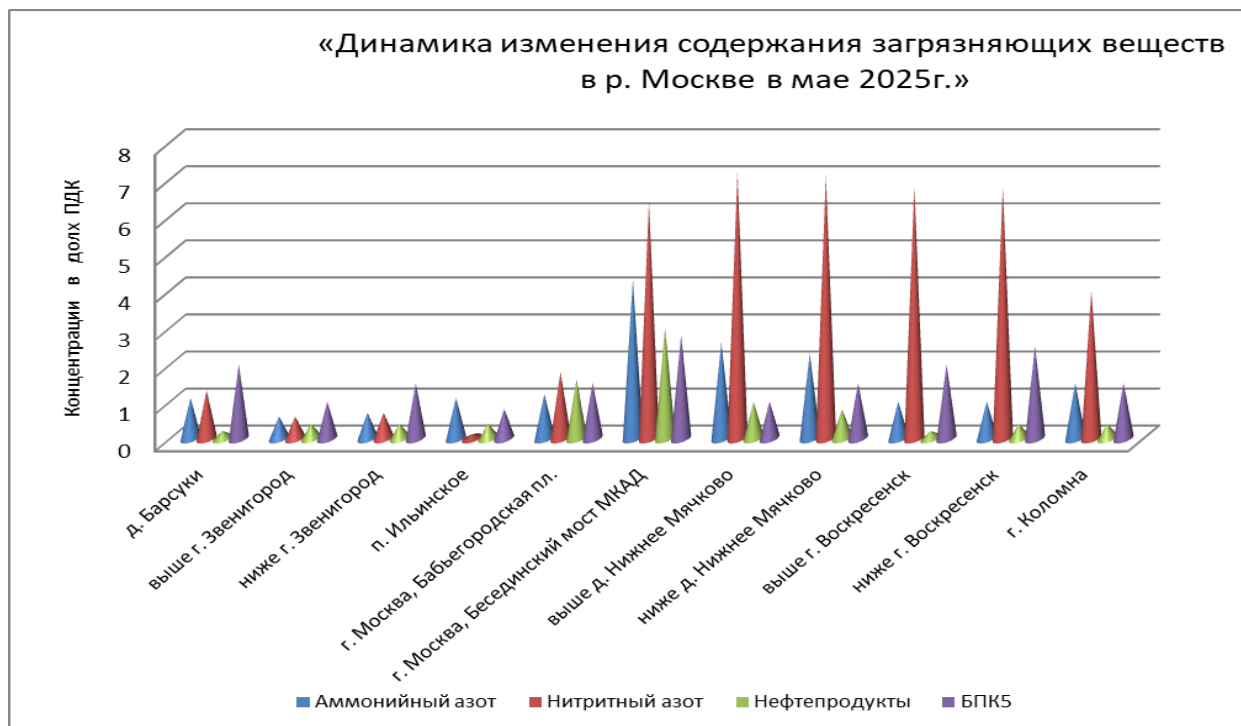
Рисунок 2 – Динамика изменения основных загрязняющих веществ в воде р. Москва в мае 2025 года (осредненные концентрации веществ в долях ПДК)
