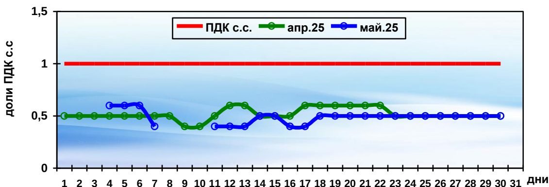
Рисунок 1 – Средние суточные концентрации диоксида азота в апреле и мае 2025 г. по данным наблюдений на стационарных постах ФГБУ «Центральное УГМС» в г. Москве
